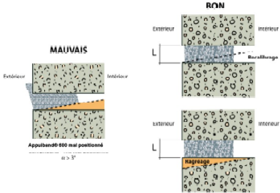
Croquis 5 - Surface de contact
