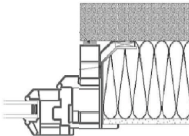
Croquis 14-3 : Exemples d'étanchéité entre tableau et menuiserie
