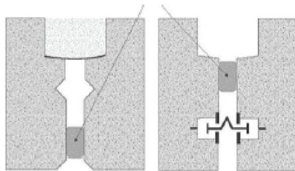
Croquis 20 : Sous-éléments préfabriqués lourds
