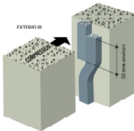
Croquis 8 : Raccords par juxtaposition des extrémités
