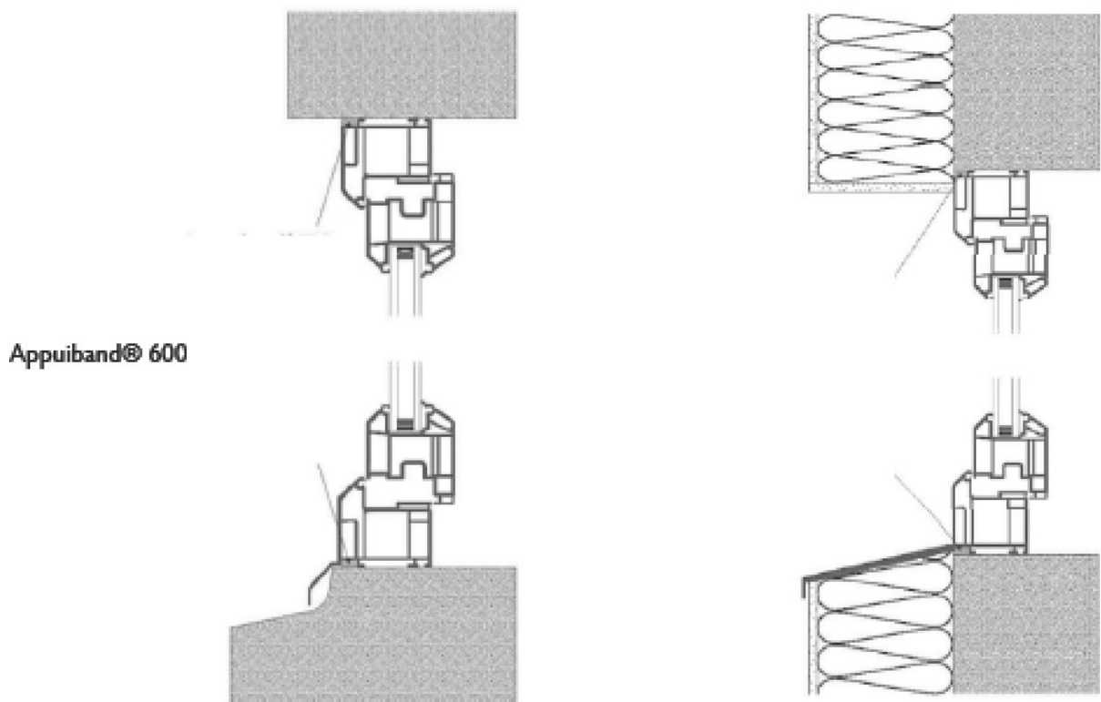
Croquis 15 : Pose en tunnel
