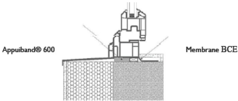
Croquis 16 : Exemple d'étanchéité sous pièce d'appui
