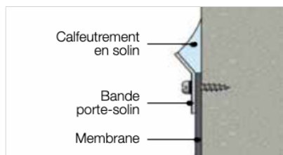
Figure 10 : Fixation avec calfeutrement complémentaire
