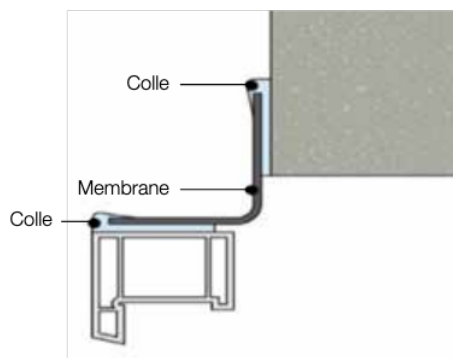
Figure 9 : Protection des plans de collage
