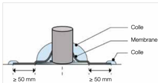
Figure 19 : Traversées diverses
