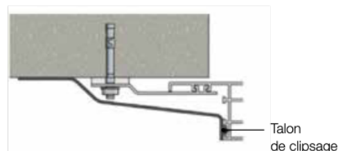
Figure 6 : Exemple de pose en façade légère avec talon de clipsage (coupe horizontale)
