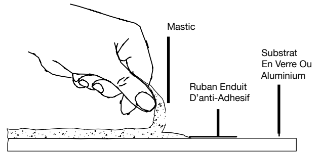
Test d'adhérence par pelage: Rupture cohésive
